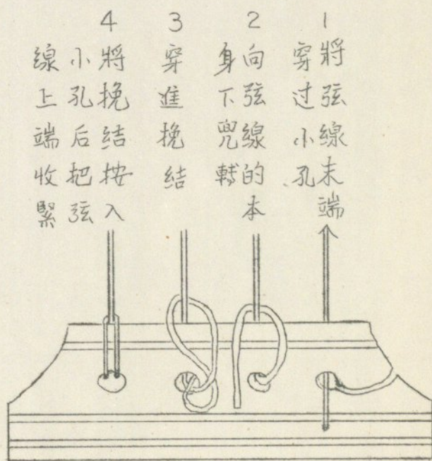
弦線靠近複手的結頭法
