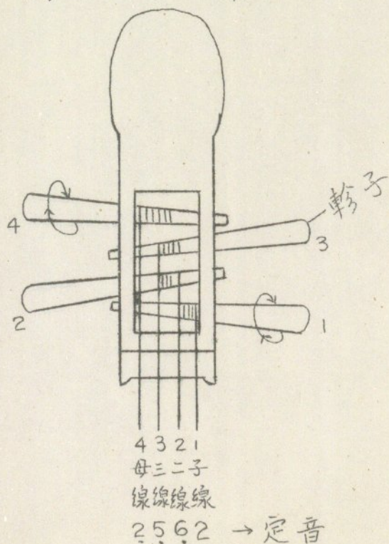
弦線與軫子排列的次序
